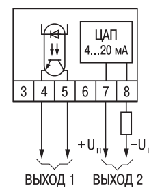
Рис. В.7. Модификация TRM202-X.KI
