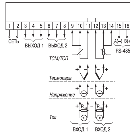
Рис. В.1. Общая схема подключения TRM202
