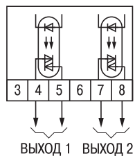
Рис. В.5. Модификация TRM202-X.CC
