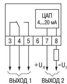
Рис. В.6. Модификация TRM202-X.PI
