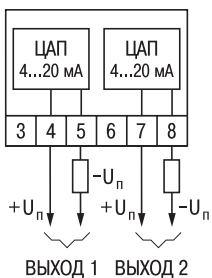
Рис. В.4. Модификация TRM202-X.II
