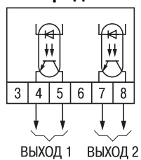
Рис. В.3. Модификация TRM202-X.KK
