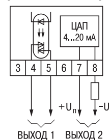
Рис. В.8. Модификация TRM202-X.SI
