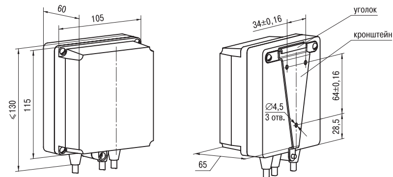
Рис. П1.1. Прибор настенного крепления
