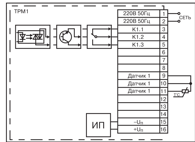
Рис. П2.1. Схема подключения термопреобразователей сопротивления
