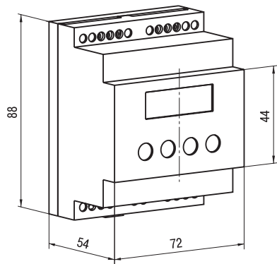
Рис. П1.4. Прибор для крепления на DIN-рейку
