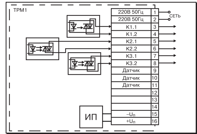
Рис. П2.5. Схема подключения прибора с трехфазным оптосимисторным выходом
