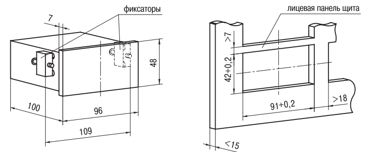
Рис. П1.3. Прибор щитового крепления Щ2
