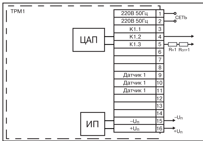
Рис. П2.6. Схема подключения прибора с аналоговым выходом 4...20 мА
