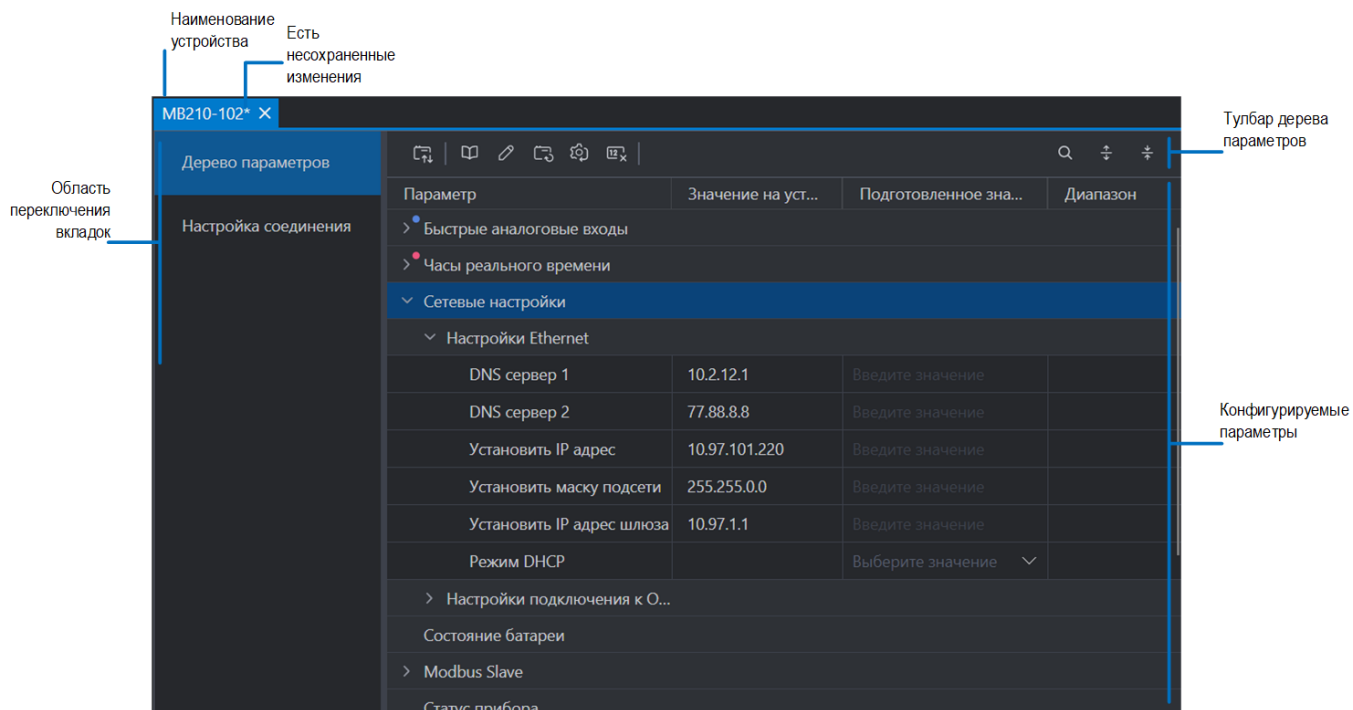
Рисунок 6.25 – Окно конфигурирования устройства
