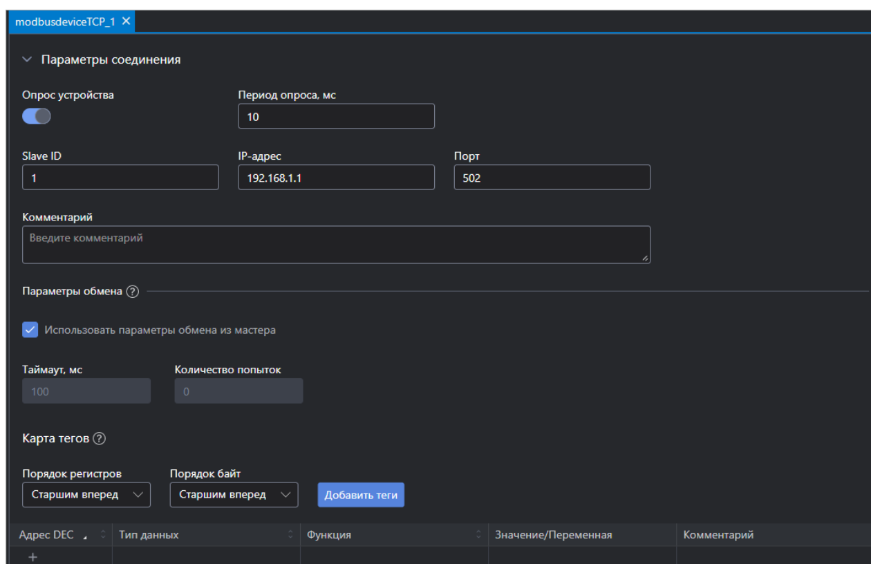
Рисунок 5.35 – Вкладка редактора Modbus Slave Device TCP
