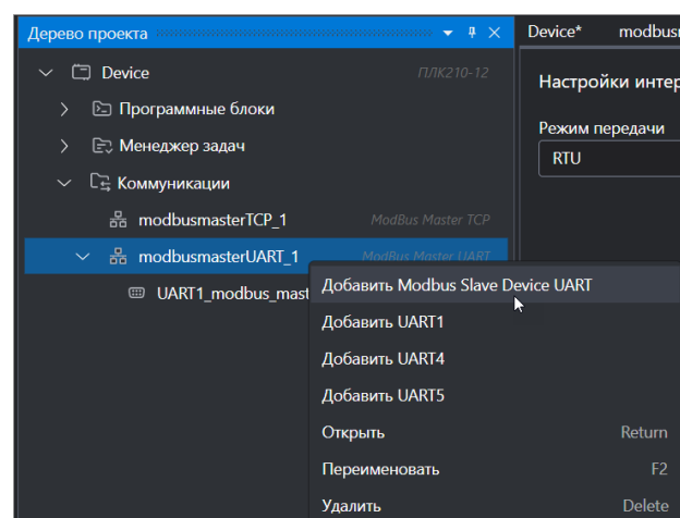
Рисунок 5.33 – Добавление Modbus Serial Slave Device
