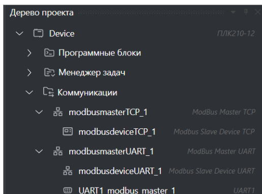
Рисунок 5.34 – Modbus Device в дереве проекта
