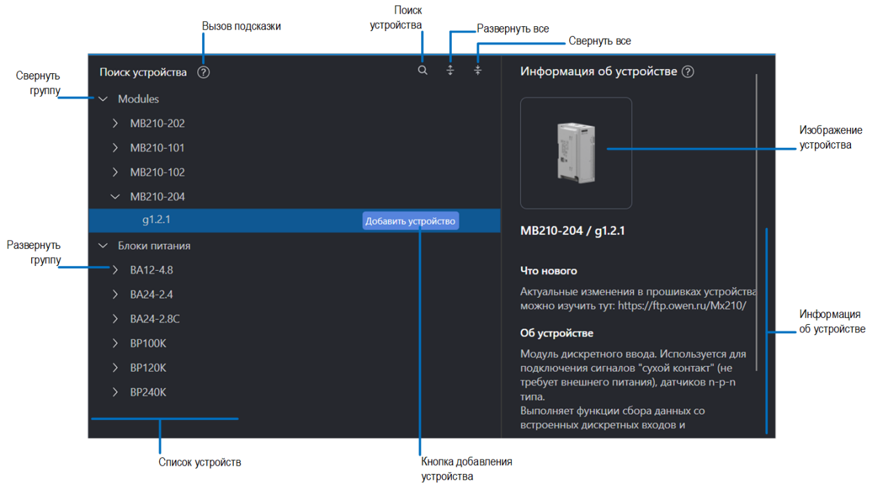
Рисунок 6.23 – Вкладка Добавить Offline
