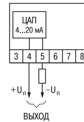
Рис. В.4. Модификация TRM201-X.I
