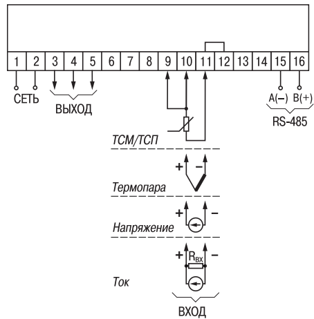
Рис. В.1. Общая схема подключения TRM201
