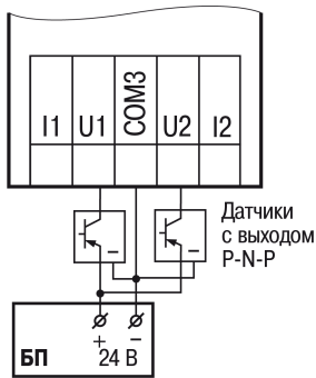
Рисунок 6.7 – Схема подключения к универсальным входам, работающим в дискретном режиме трехпроводных дискретных датчиков, имеющих выходной транзистор р-п-р-типа с открытым коллектором
