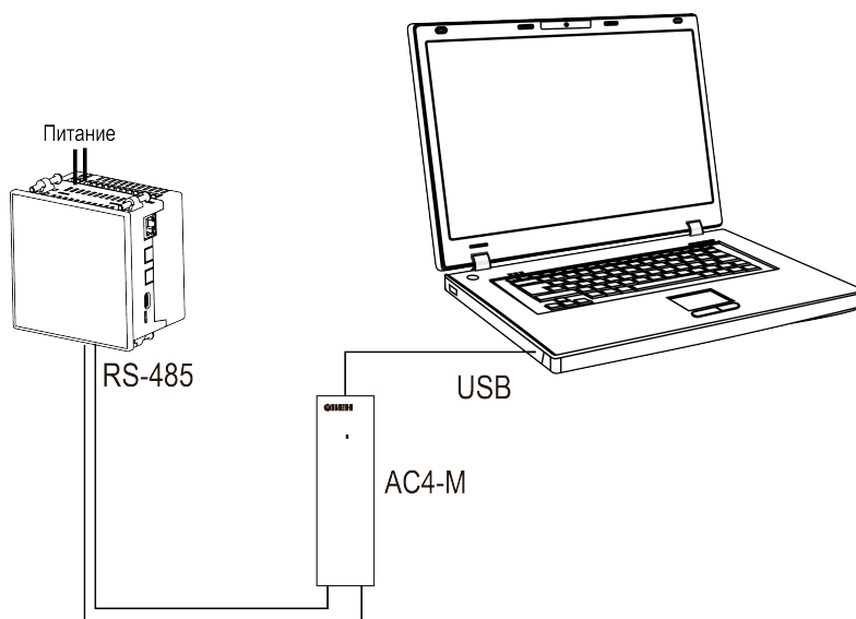
Рисунок 6.22 – Схема подключения прибора к ПК по RS-485
