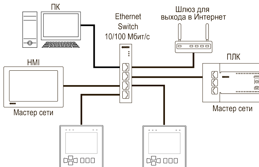
Рисунок 6.18 – Подключение по схеме «Звезда»
