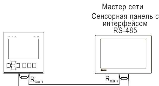
Рисунок 6.16 – Типовая схема подключения в режиме Slave
