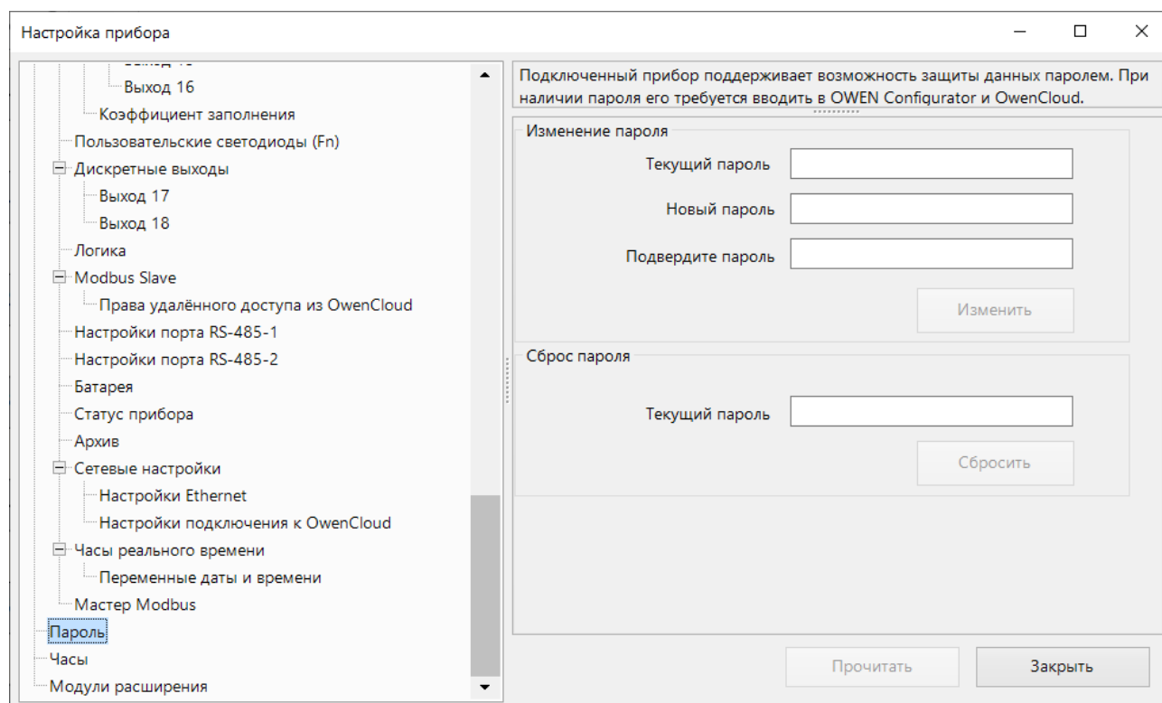
Рисунок 4.17 – Пароль доступа
