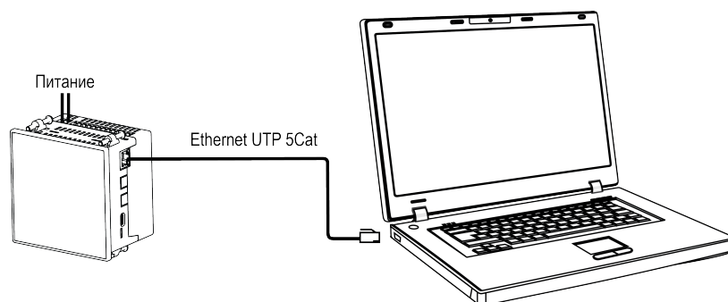
Рисунок 6.21 – Схема подключения прибора к ПК по Ethernet
