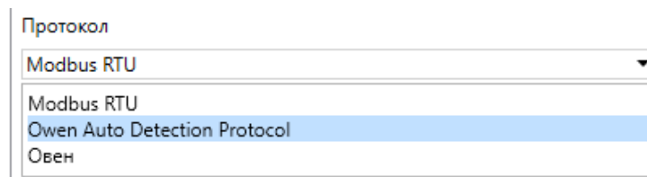
Рисунок 4.16 – Выбор протокола
