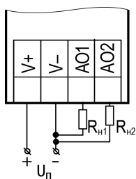
Рисунок 6.13 – Подключение аналогового выхода, находящегося в режиме источника тока
