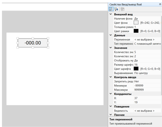
Рисунок 7.143 – Ввод/вывод float
