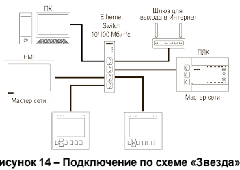
Рисунок 14 – Подключение по схеме «Звезда»
