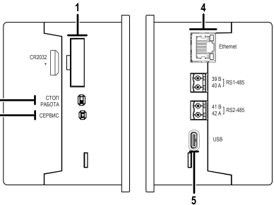
Рисунок 18 – Описание боковых поверхностей
