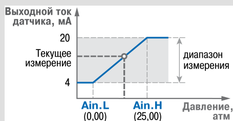
Рисунок 10.6 – Пример задания диапазона измерения
