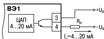
Рисунок 5.11 – Подключение нагрузки к ВЭ типа «И»
