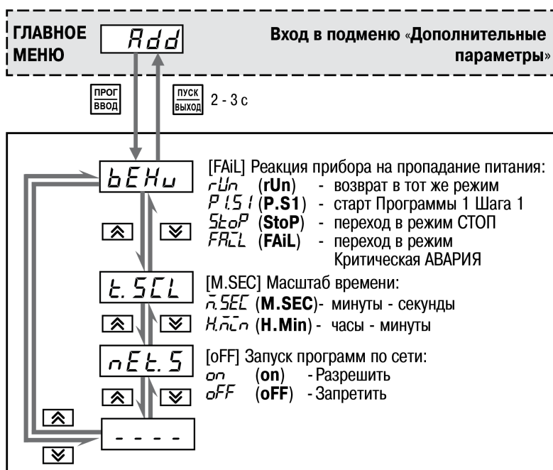
Рисунок 8.10 – Дополнительные параметры
