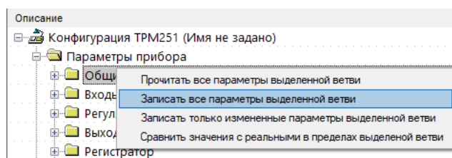
Рисунок 9.2 – Контекстное меню
