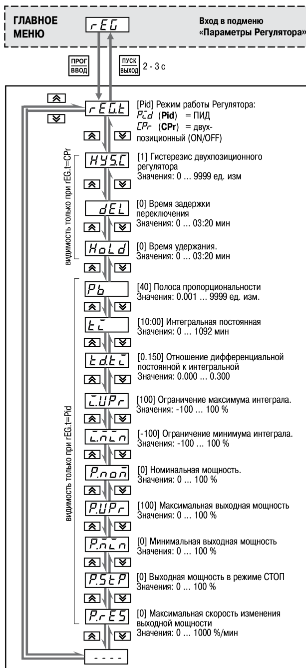
Рисунок 8.3 – Параметры регулятора
