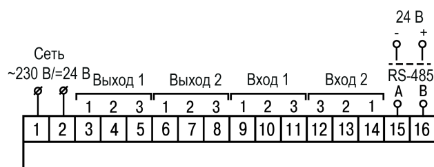
Рисунок 5.7 – Общая схема подключения 2TRM1–Н
