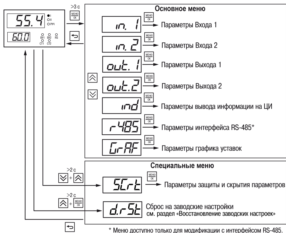
Рисунок 7.1 – Структура меню
