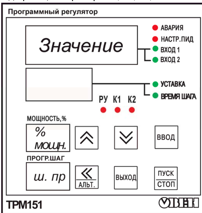
Рисунок 6.3 – Вариант 2 индикации прибора
