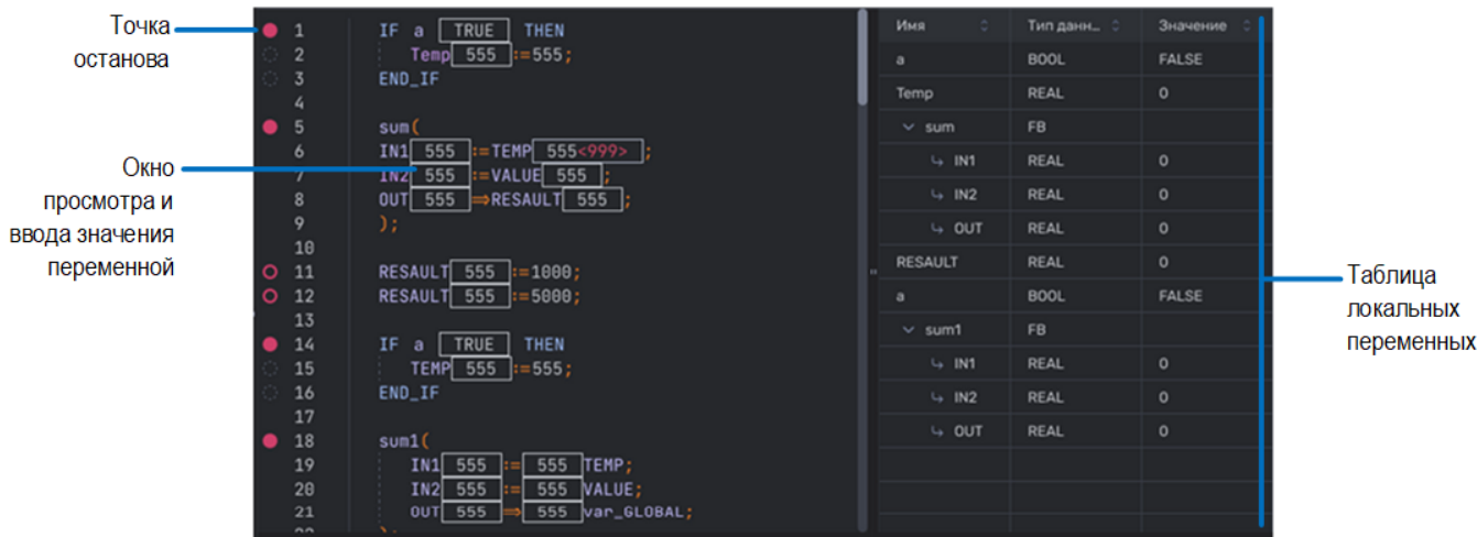
Рисунок 5.18 – Редактор ST в режиме онлайн
