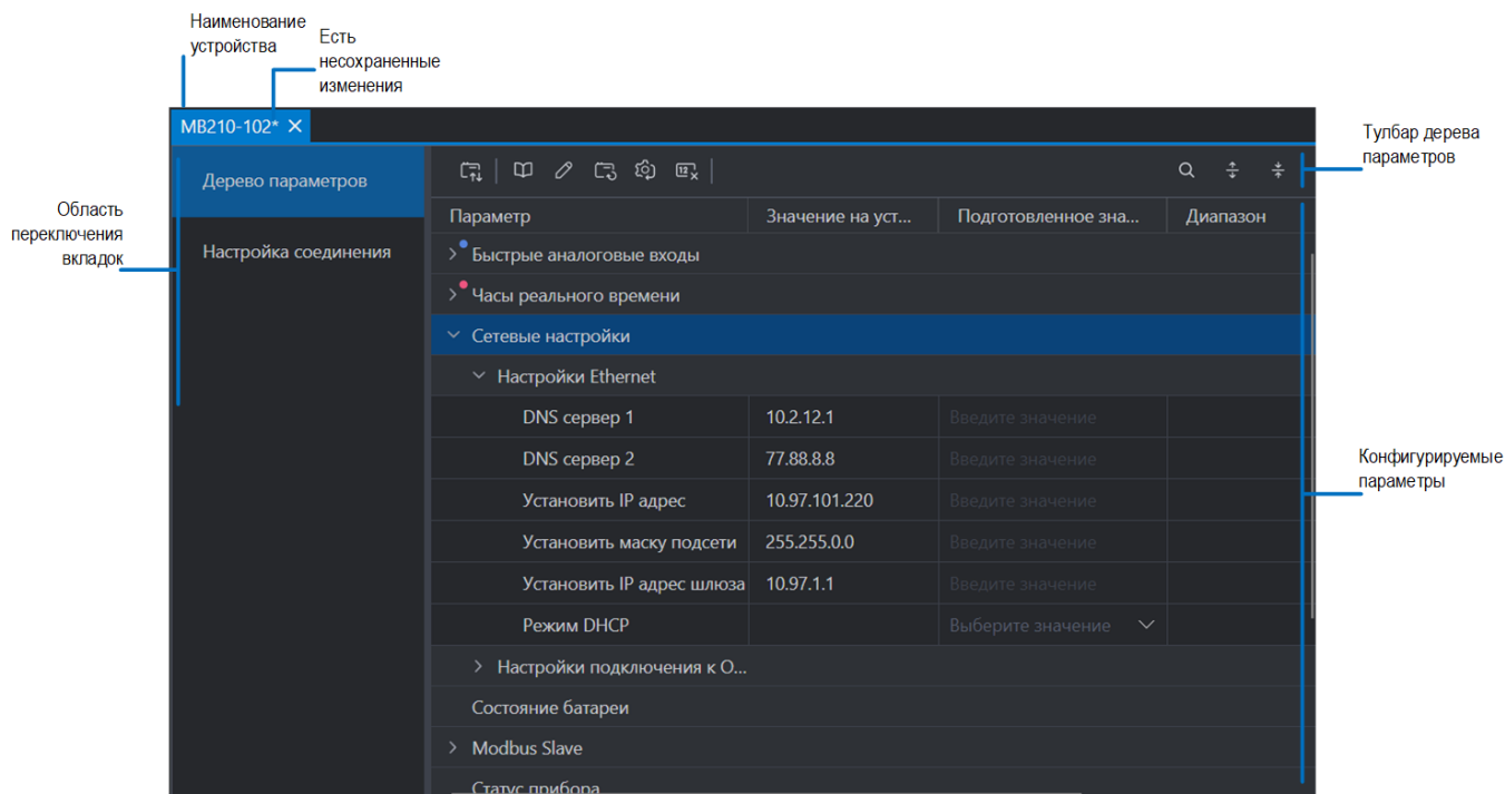
Рисунок 6.23 – Окно конфигурирования устройства
