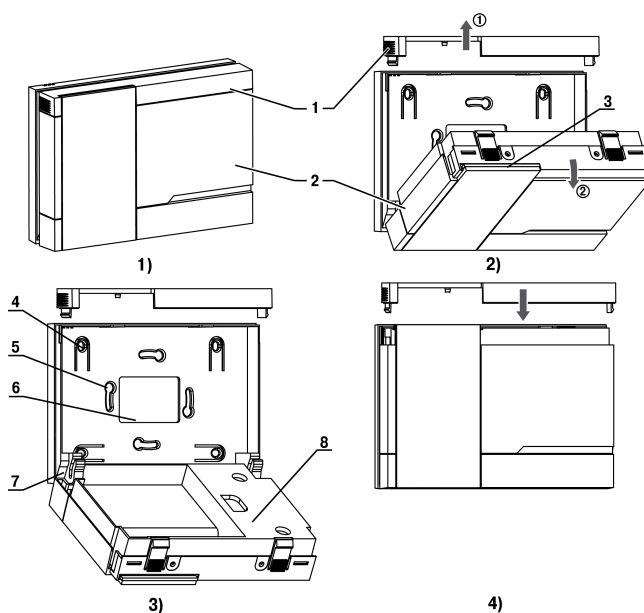
Рисунок 4.3 – Монтаж прибора настенного исполнения H2
