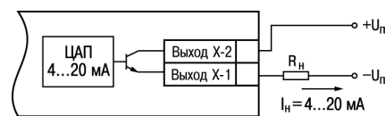
Рисунок 5.16 – Подключение к ВУ типа И
