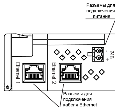
Рисунок 4 – Разъемы прибора
