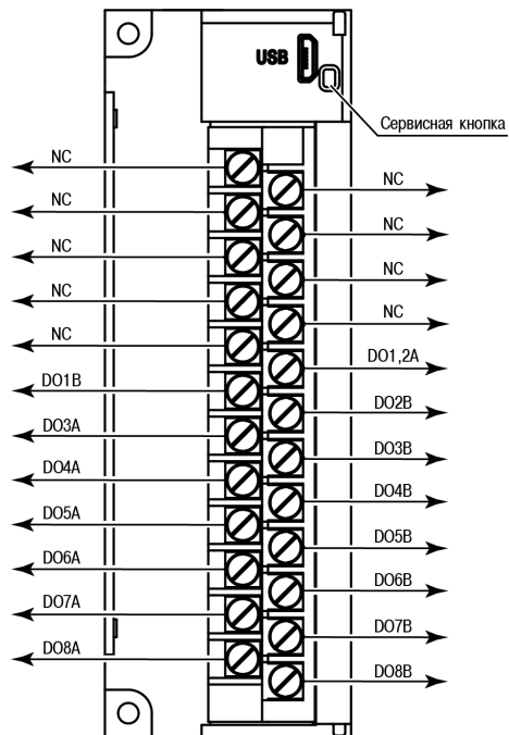
Рисунок 1 – Назначение контактов клеммника
