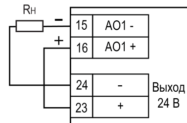
Рисунок 7.11 – Подключение выхода типа И с питанием от ИП24
