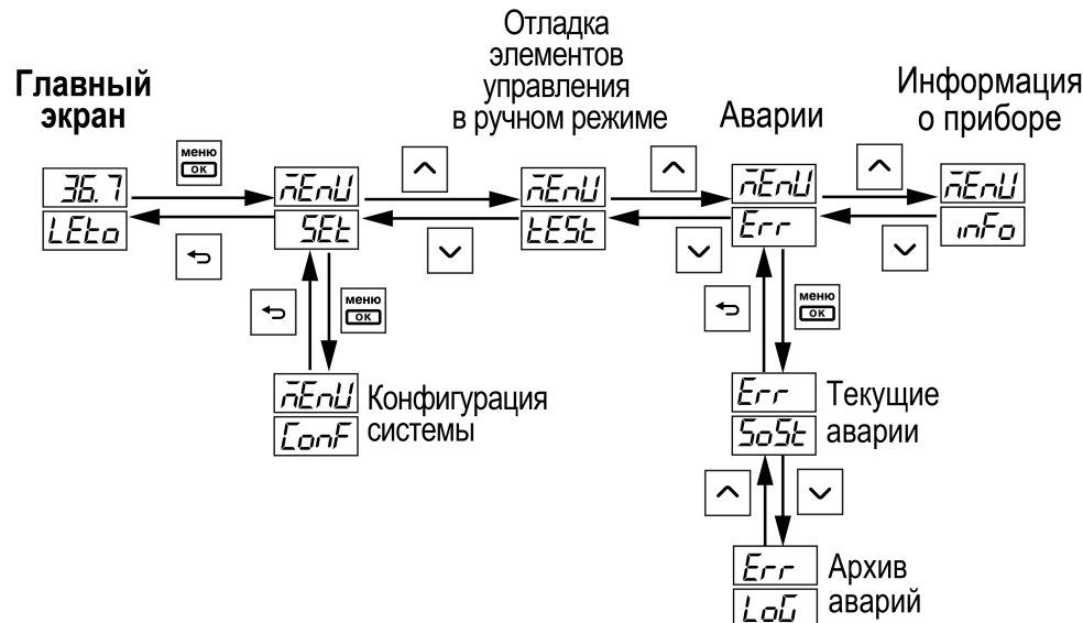
Рисунок 8.3 – Структура меню
