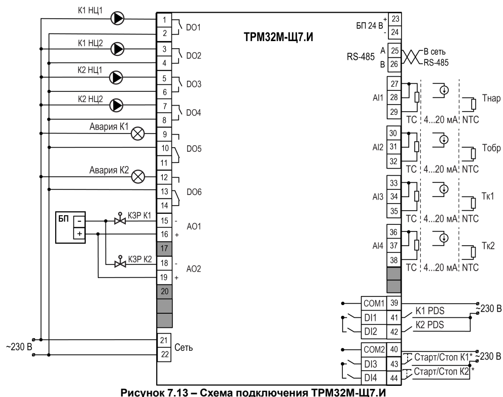
Рисунок 7.13 – Схема подключения ТРМ32М-Ц7.И
