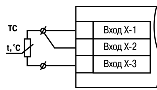
Рисунок 7.8 – Трехпроводная схема подключения ТС
