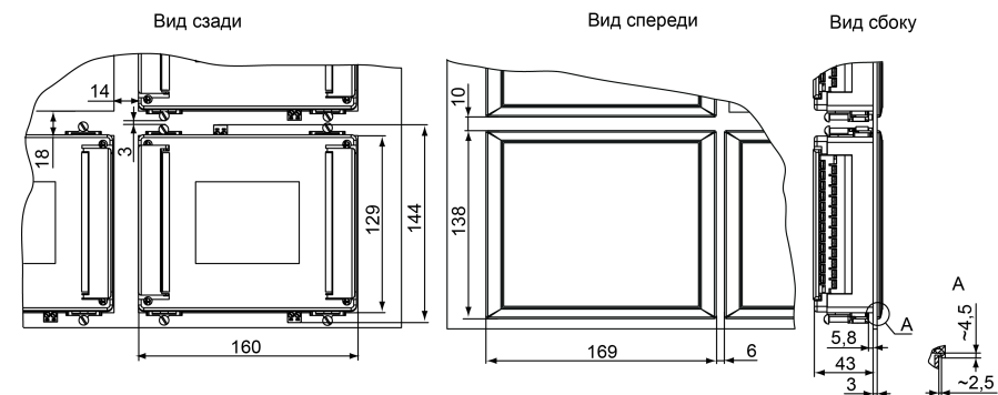
Рисунок 7.3 – Прибор в корпусе Щ7, установленный в щит толщиной 3 мм
