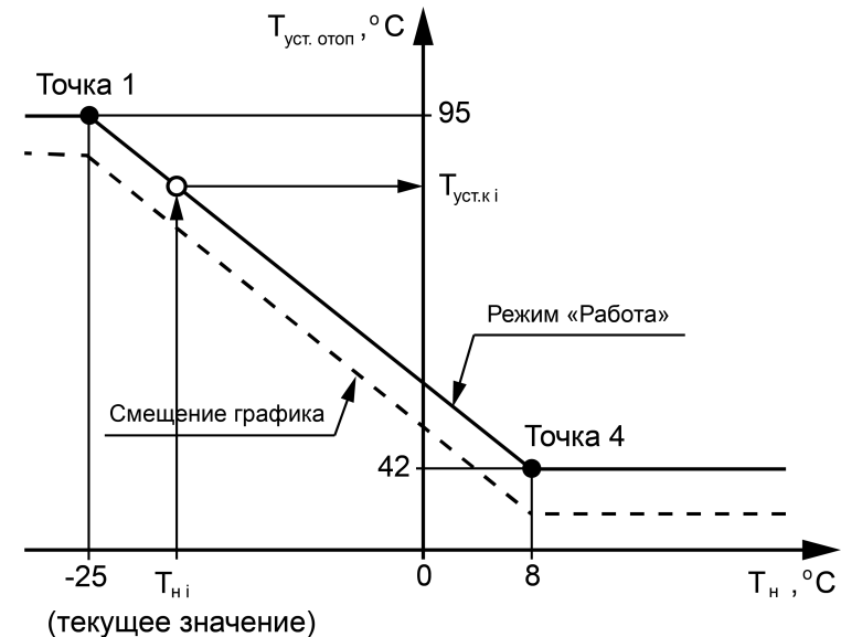
Рисунок 10.2 – Отопительный график
