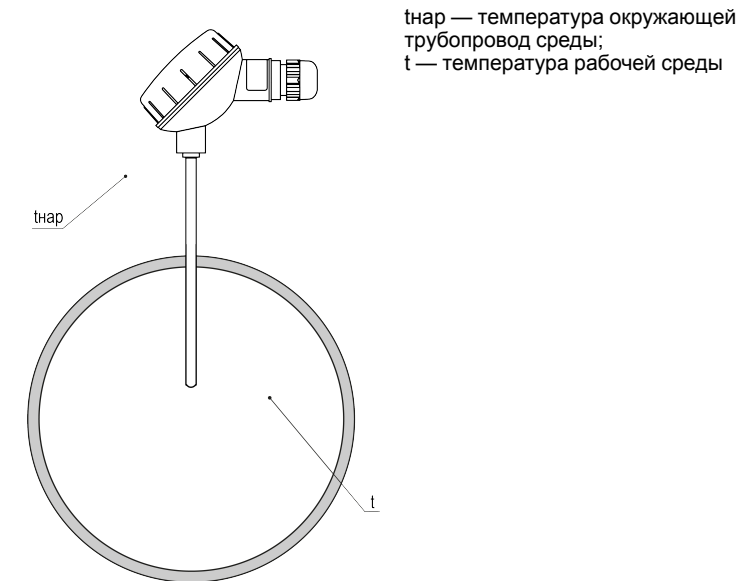
Рисунок А.6 – Пример неверного монтажа датчика
