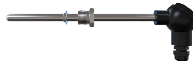
Рисунок А.3 – ДТСxx5 с подвижным штуцером (модели 035, 045, 145 и 335)
