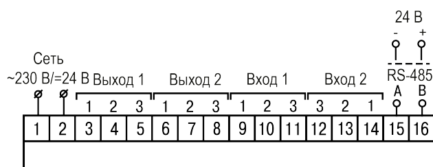
Рисунок 5.7 – Общая схема подключения TRM12–Н
