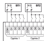
Рисунок 4 – Схема подключения дискретных датчиков с питанием 24 В к входам типа «Д»
