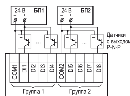
Рисунок 3 – Схема подключения к дискретным входам трехпроводных дискретных датчиков, имеющих выходной транзистор p-n-p-типа с открытым коллектором для сигналов 24 В
