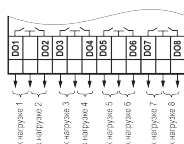
Рисунок 9 – Схема подключения к выходам типа «Р»
