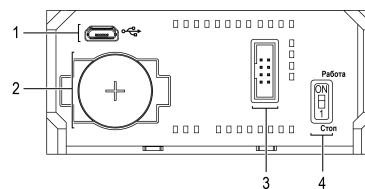
Рисунок 9 – Лицевая панель под крышкой
