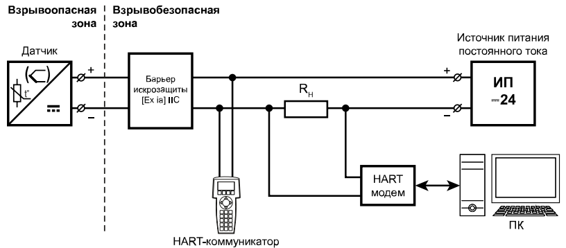
Рисунок 6 – Пример системы с HART-коммуникатором
