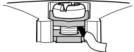
Рисунок 4 – Монтаж провода
