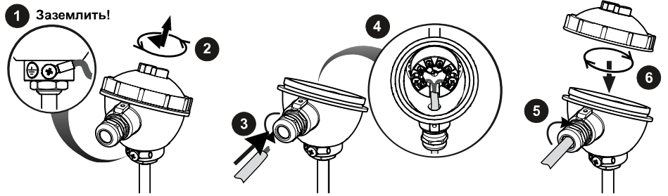
Рисунок 3 – Монтаж внешних электрических цепей
