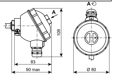
Рисунок 1 – Габаритный чертеж коммутационной головки
