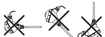
Рисунок 1 – Положения датчика при монтаже
