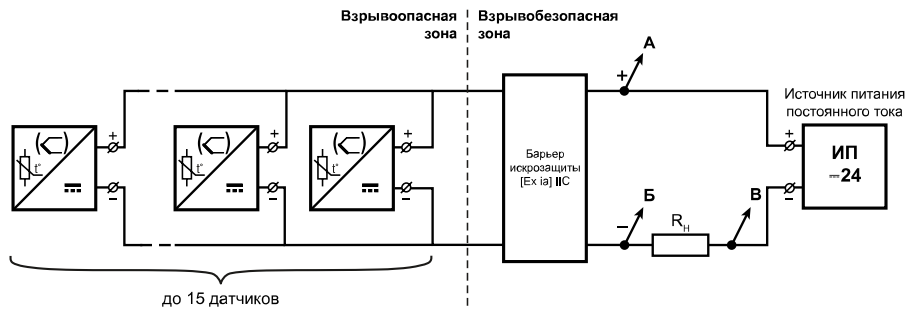
Рисунок 7 – Пример системы с параллельным подключением датчиков
