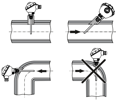
Рисунок 2 – Монтаж датчика на объекте
