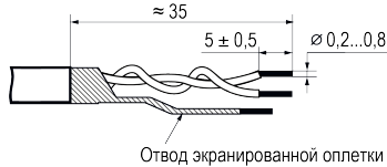
Рисунок 5.1 – Подготовка кабеля
