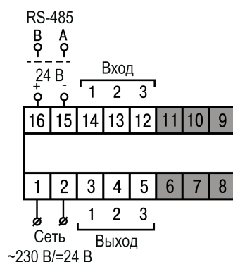
Рисунок 5.5 – Общая схема подключения ТРМ1–Ц5
