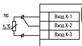
Рисунок 5.15 – Трехпроводная схема подключения ТС
