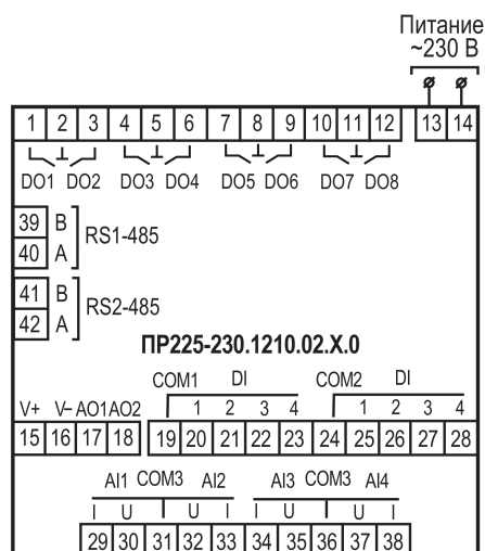
Рисунок А.3 – Расположение контактов для ПР225–230.1210.02.X.0
