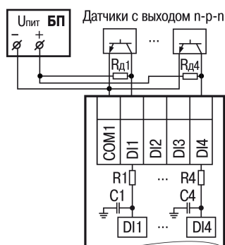
Рисунок 6.12 – Подключение к входам типа «Д» датчиков с выходом n-p-n
