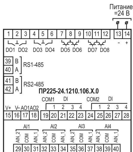
Рисунок А.15 – Расположение контактов для PR225–24.1210.106.X.0
