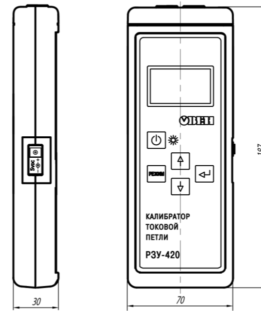
Рисунок 4 – Габаритный чертёж прибора
