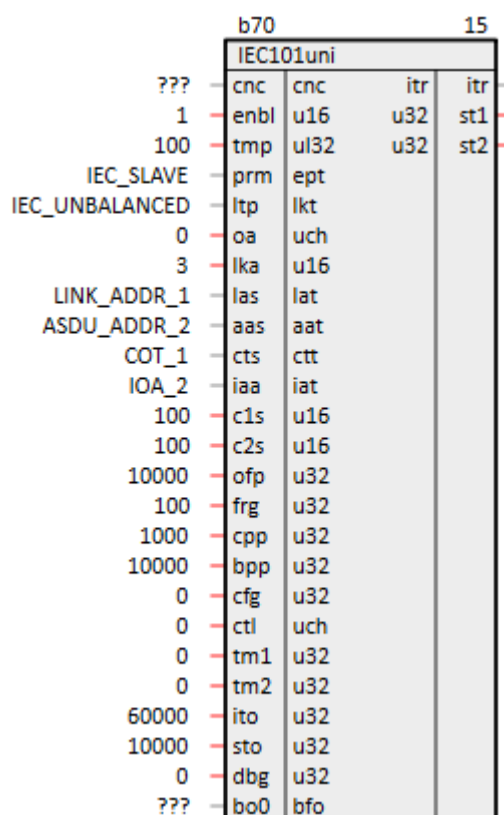
Рисунок 2.4 – Блок IEC101uni
