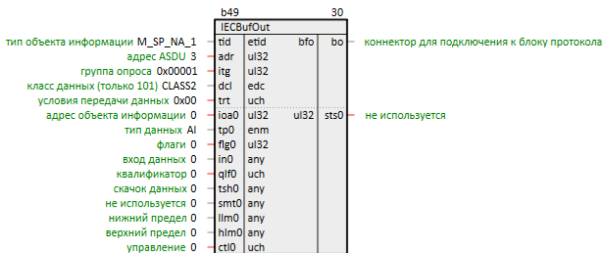
Рисунок 2.10 – Блок IECBufOut
