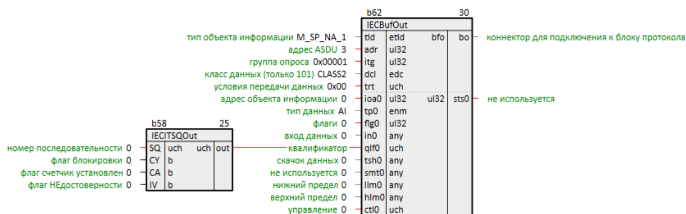
Рисунок 2.14 – Блок IECITSQOut
