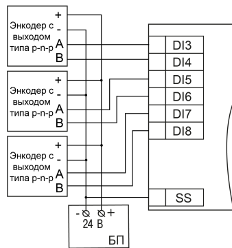
Рисунок 6 – Подключение энкодеров р-п-п
