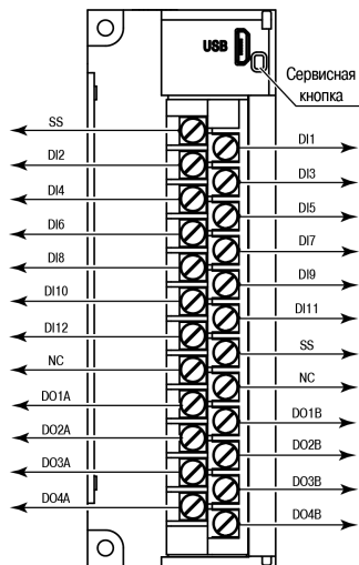
Рисунок 1 – Назначение контактов клемника
