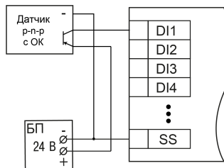
Рисунок 4 – Подключение транзисторов р-п-п
