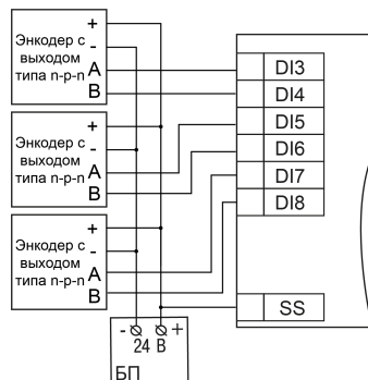
Рисунок 7 – Подключение энкодеров п-р-п
