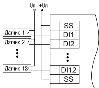
Рисунок 3 – Схема подключения к входам DI1 – DI12
