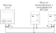
Рисунок 10 – Типовая схема подключения в режиме Master
