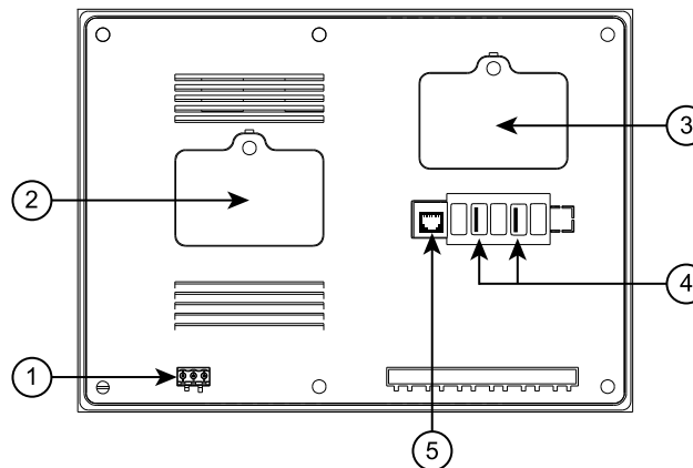
Рисунок 5 – Внешний вид задней стороны прибора
