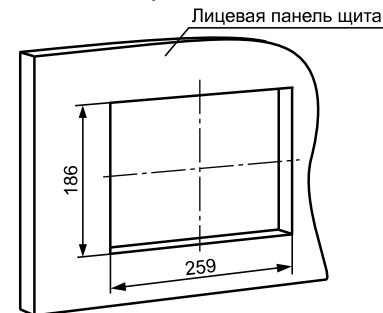
Рисунок 2 – Установочные размеры для крепления в щит
