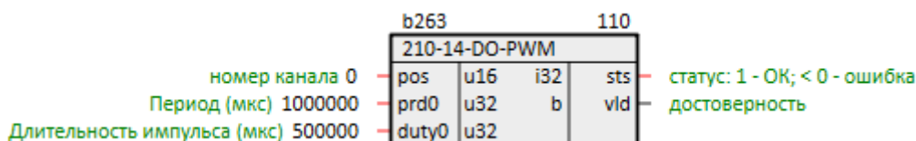
Рисунок 1.31 – ШИМ дискретных выходов DO 1...4 (210-14-DO-PWM)
