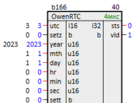
Рисунок 2.4 – Работа OwenRTC
