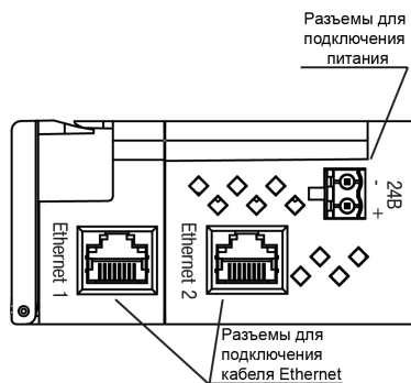
Рисунок 2 – Разъемы прибора
