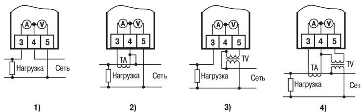
Рисунок 5.2 – Подключение: 1) к однофазной сети, 2) к однофазной сети через согласующий трансформатор тока, 3) к однофазной сети через согласующий трансформатор напряжения, 4) к однофазной сети через согласующие трансформаторы тока и напряжения
