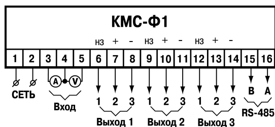
Рисунок 5.1 – Назначение клеммника
