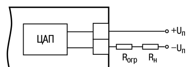
Рисунок 5.7 – Схема соединения ЦАП с нагрузкой
