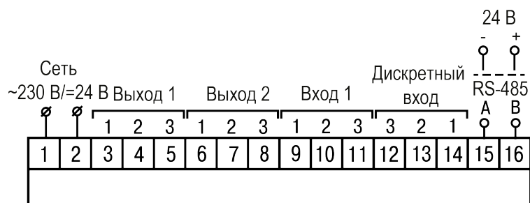
Рисунок 5.7 – Общая схема подключения TPM10–Н
