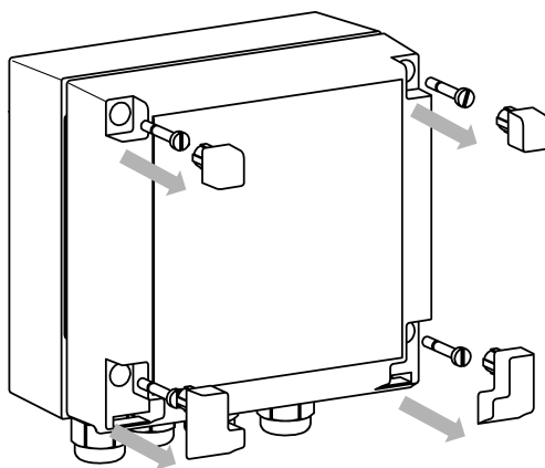
Рисунок 4.12 – Разборка передней части корпуса
