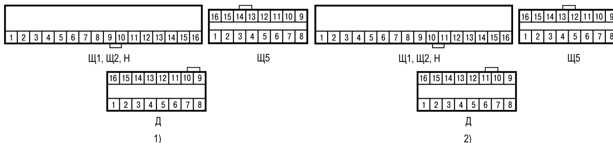
Рисунок 7.8 – Установка переключки
