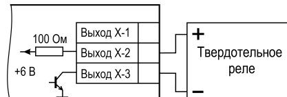
Рисунок 5.25 – Схема подключения нагрузки к ВУ типа «Т»
