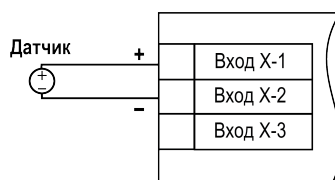
Рисунок 5.20 – Схема подключения активного датчика с выходными сигналами напряжения постоянного тока от 0 до 5 В и от 0 до 10 В
