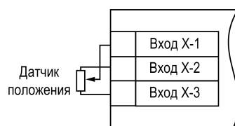
Рисунок 5.22 – Подключение датчика положения резистивного типа
