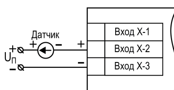
Рисунок 5.21 – Схема подключения пассивного датчика с выходным сигналом силы постоянного тока от 0 до 5 мА или от 0(4) до 20 мА
