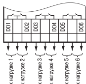
Рисунок 9 – Схема подключения ВЭ типа «Р»
