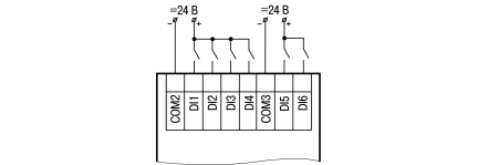
Рисунок 3 – Подключение к дискретным входам датчиков типа «сухой контакт» для сигналов =24 В
