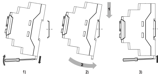
Рисунок 2 – Монтаж прибора
