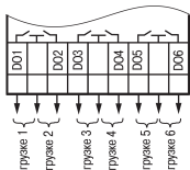
Рисунок 10 – Схема подключения ВЭ типа «Р»
