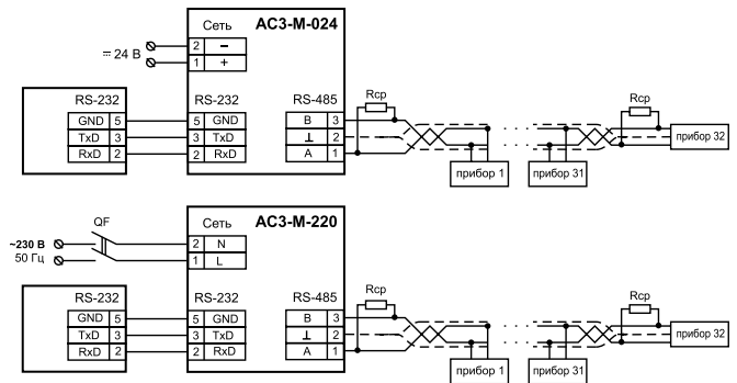
Рисунок 5 – Схемы подключения
