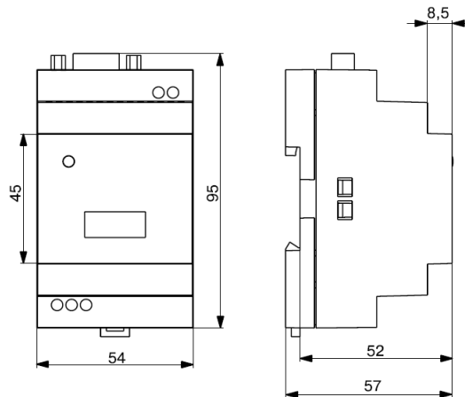
Рисунок 1 – Габаритный чертеж
