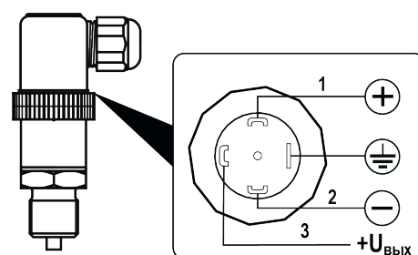
Рисунок 6.4 – Маркировка контактов соединителя
