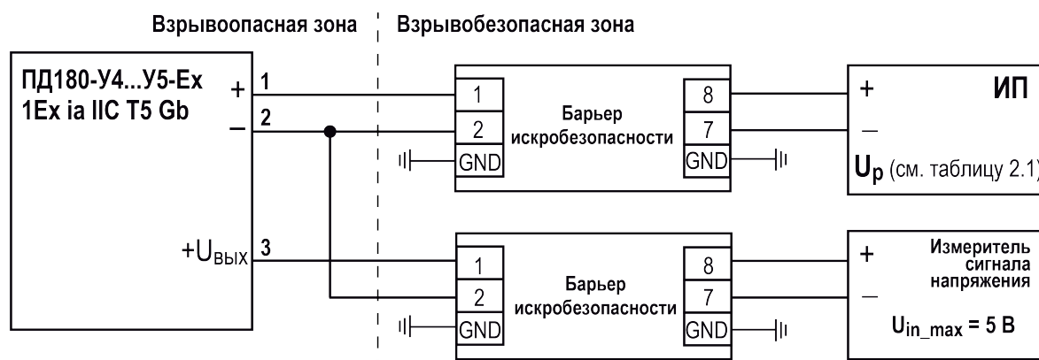
Рисунок 6.7 – Схема подключения ПД180-У4...У5-Ех во взрывоопасной зоне через барьер искробезопасности
