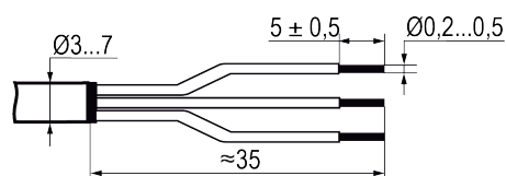
Рисунок 6.2 – Подготовка кабеля
