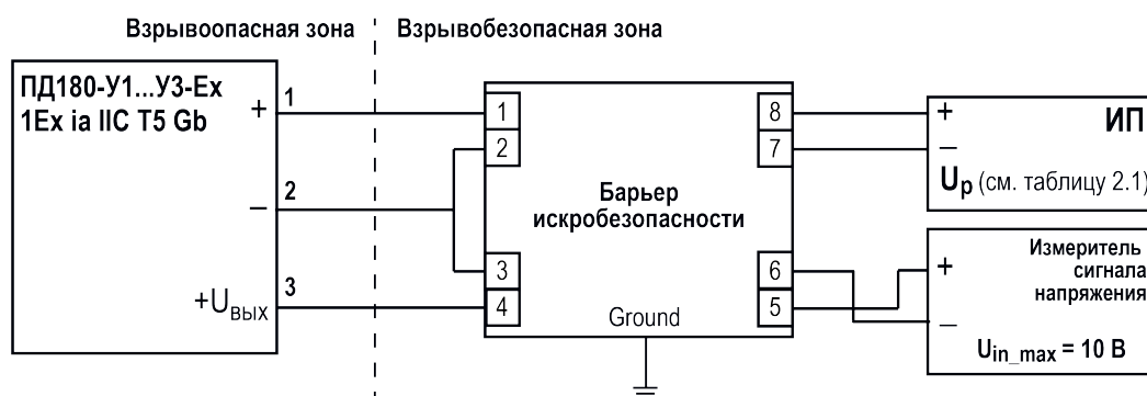
Рисунок 6.6 – Схема подключения ПД180-У1...У3-Ех во взрывоопасной зоне через барьер искробезопасности
