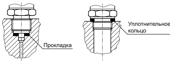
Рисунок 5.2 – Варианты уплотнения
