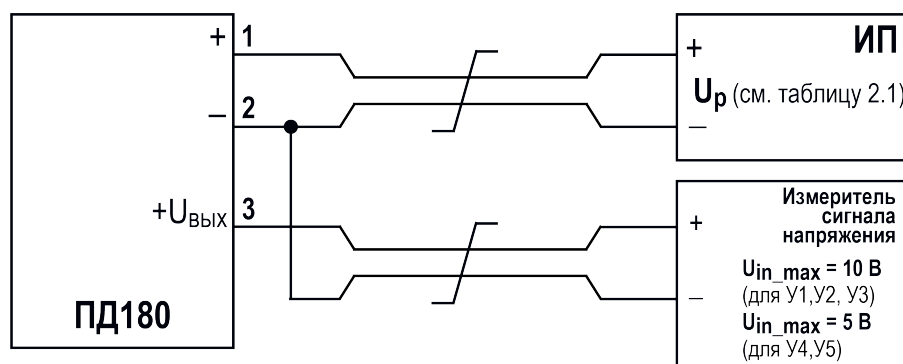
Рисунок 6.5 – Схема подключения преобразователя в общепромышленном исполнении
