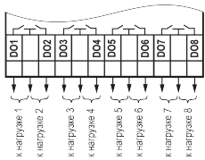
Рисунок 8 – Схема подключения к выходам типа «Р»
