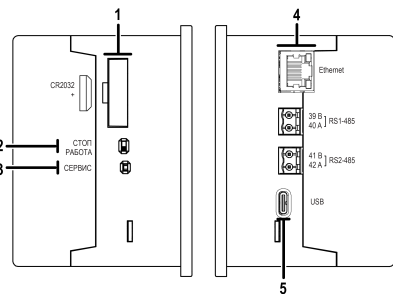
Рисунок 16 – Описание боковых поверхностей
