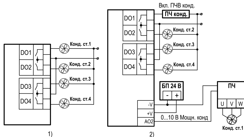
Рисунок 7.9 – Схема подключения на примере конфигурации из 4-х ступеней конденсатора без компрессоров, где 1-я ступень управляется: 1) дискретно вкл/откл; 2) с помощью ПЧ
