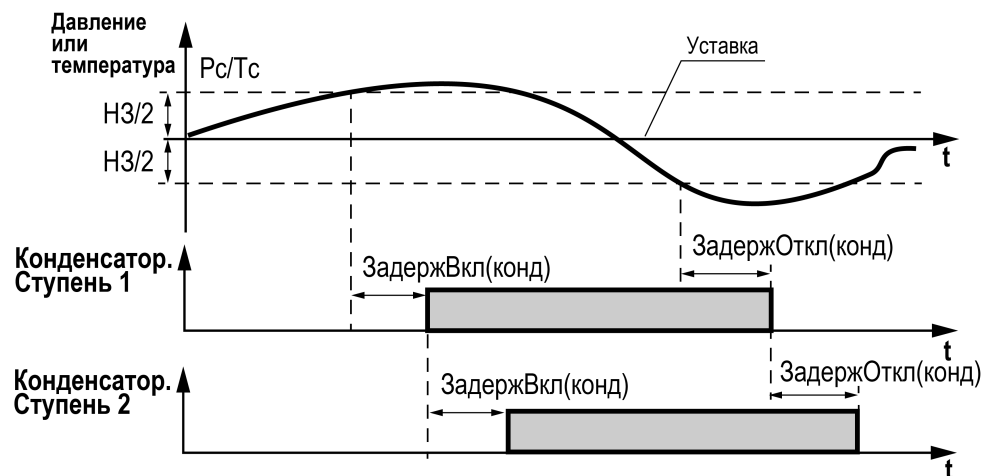
Рисунок 8.8 – Диаграмма регулирования с нейтральной зоной на примере 2-х ступеней конденсатора
