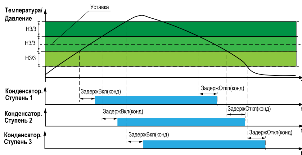
Рисунок 8.9 – Диаграмма регулирования с зонами пропорциональности на примере 3-х ступеней конденсатора
