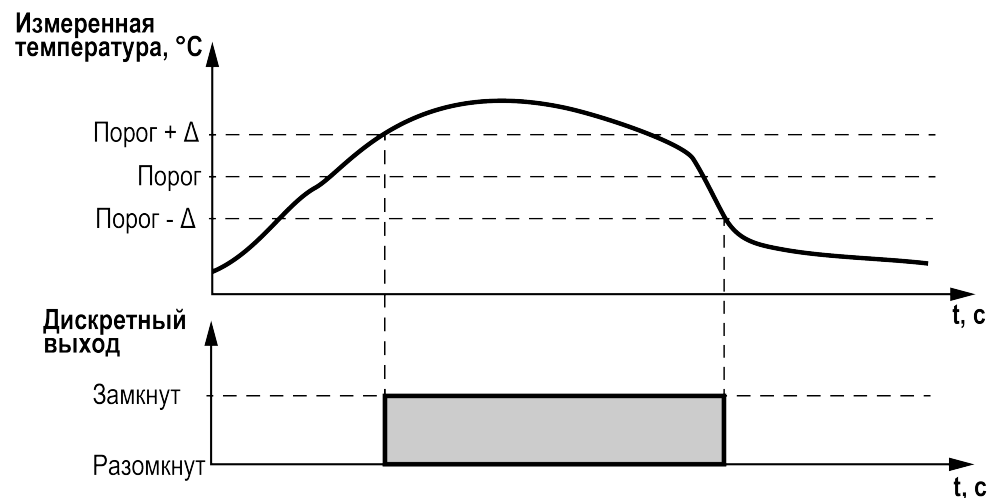
Рисунок 8.13 – Иллюстрация работы функции «Независимый термостат»
