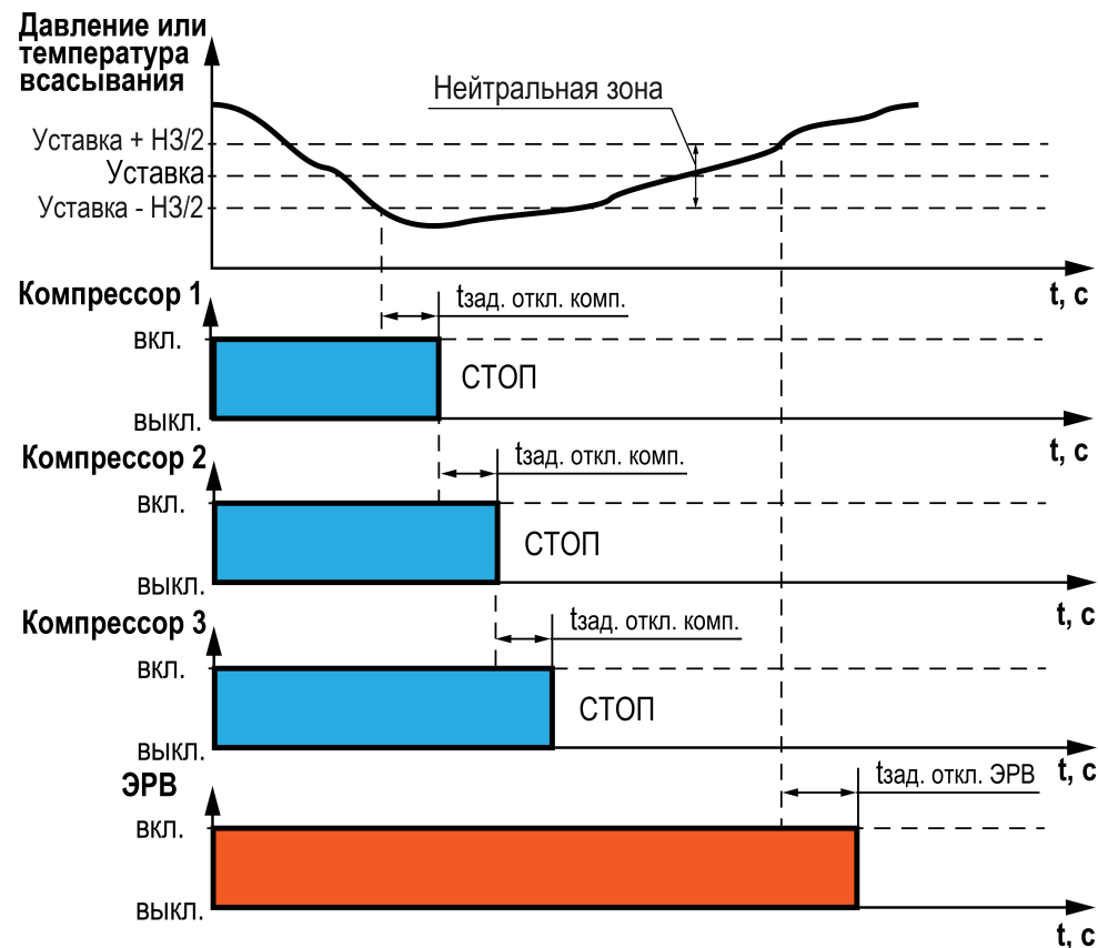
Рисунок 8.14 – Иллюстрация работы функции «Антизалив» компрессоров
