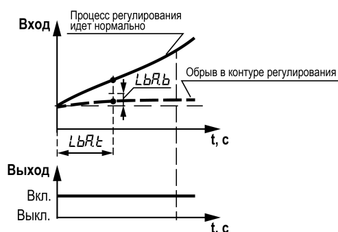
Рисунок 7.4 – Диагностика обрыва в контуре регулирования
