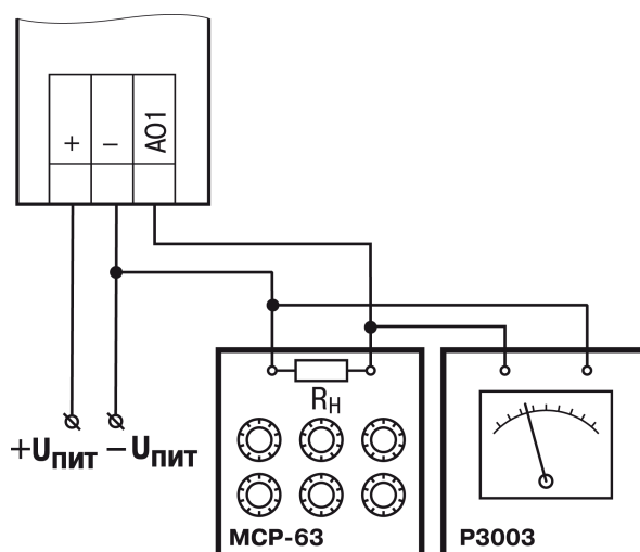
Рисунок В.3 – Схема подключения к ВЭ для юстировки сигналов типа «4...20 мА» ( R_H < 600 Ом)
