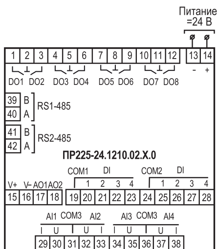
Рисунок А.7 – Расположение контактов для ПР225–24.1210.02.X.0
