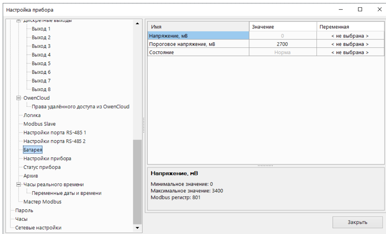
Рисунок 4.36 – Параметры состояния батареи
