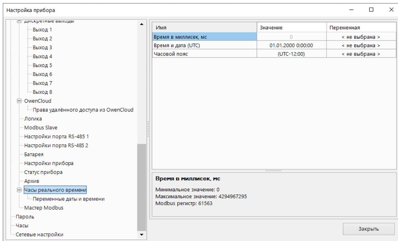
Рисунок 4.32 – Привязка переменных к настройкам часов реального времени
