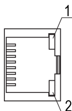
Рисунок 7.4 – Расположение светодиодов порта Ethernet: 1) зеленый, 2) оранжевый
