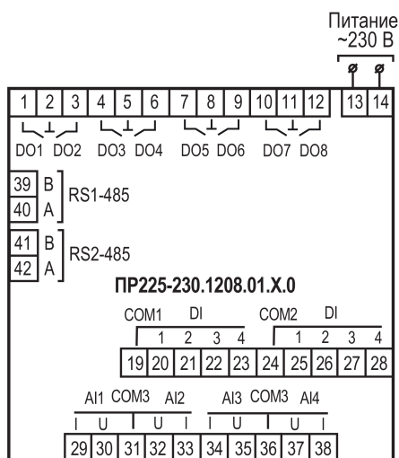
Рисунок А.2 – Расположение контактов для ПР225–230.1208.01.X.0
