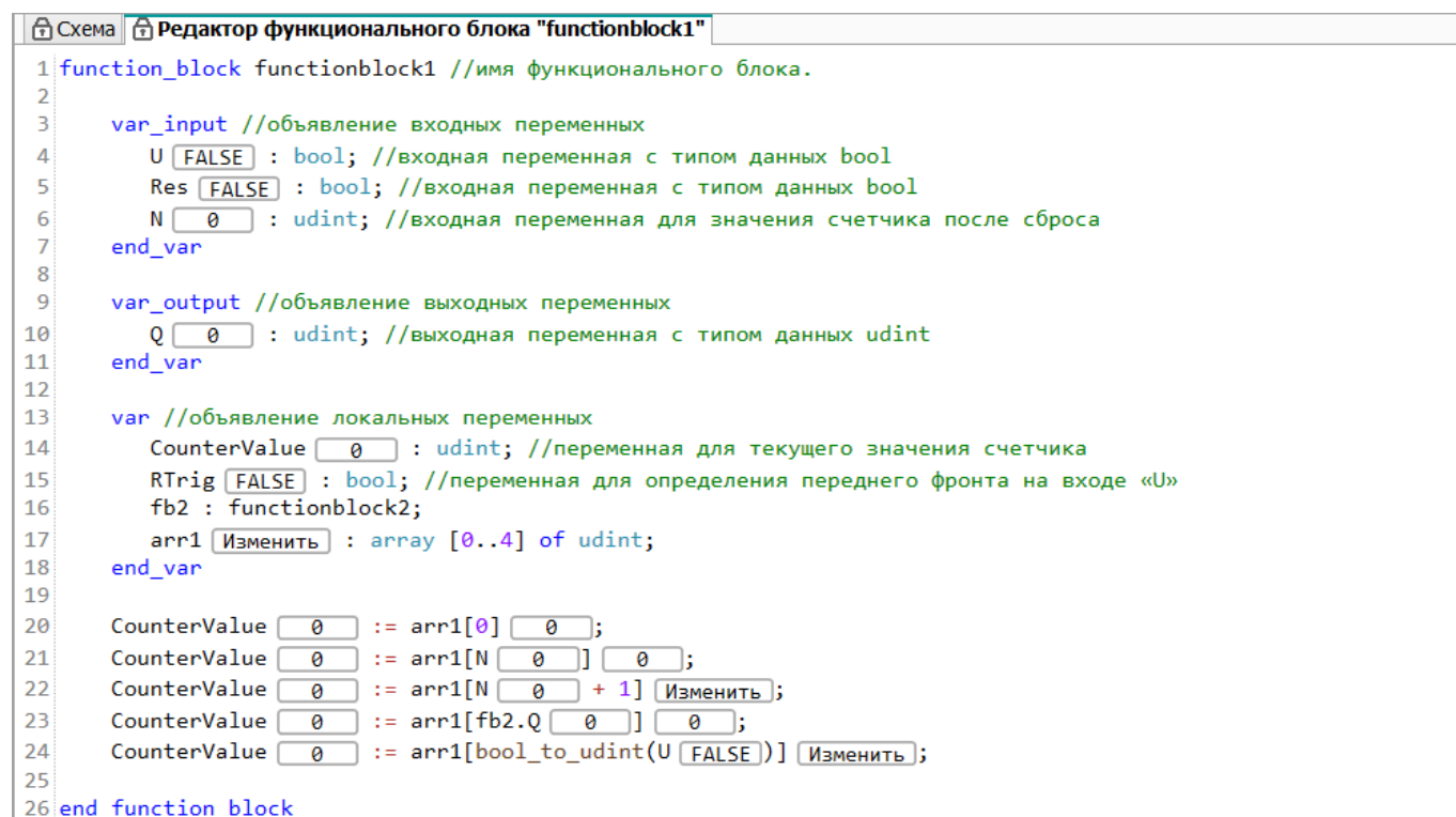
Рисунок 4.85 – Окно Редактор функционального блока в режиме симулятора
