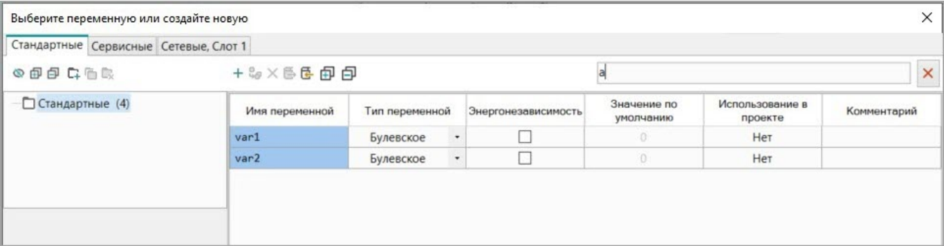
Рисунок 6.5 – Поиск переменных
