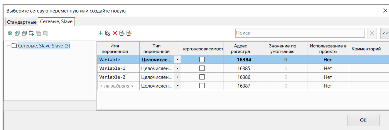
Рисунок 5.46 – Таблица переменных
