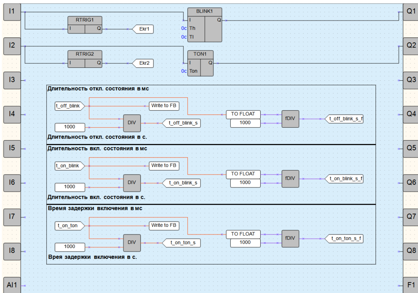
Рисунок 11.5 – Схема алгоритма
