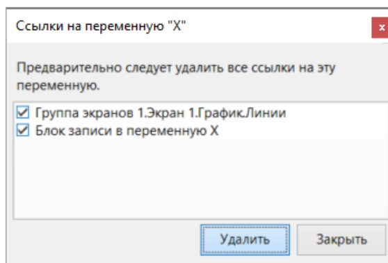
Рисунок 7.168 – Информационное окно
