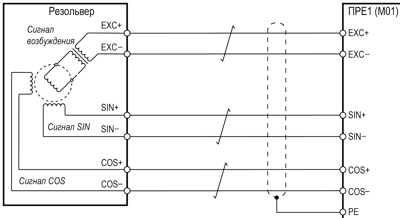
Рисунок 8.17 – Схема подключения резольвера
