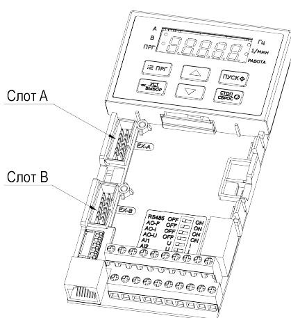
Рисунок 8.4 – Расположение разъемов для подключения плат расширения
