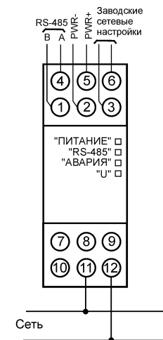
Рисунок 1 – Подключение прибора к однофазной сети
