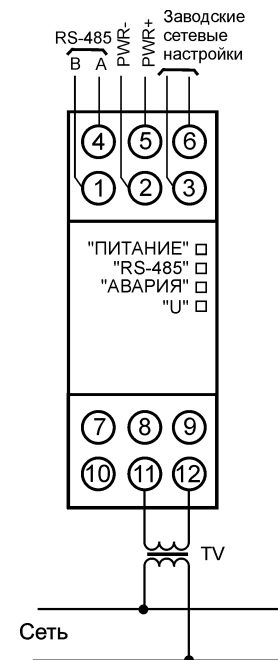
Рисунок 2 – Подключение прибора к однофазной сети через согласующий трансформатор
