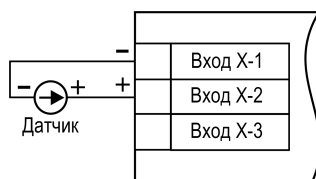
Рисунок 5.12 – Схема подключения пассивного датчика с выходным сигналом силы постоянного тока от 0 до 5 мА или от 0(4) до 20 мА с питанием от прибора
