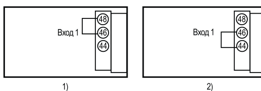
Рисунок 7.8 – Установка перемычки
