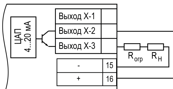
Рисунок 5.5 – Подключение выхода типа И с питанием от ИП24
