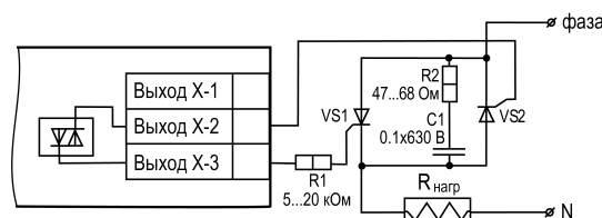
Рисунок 5.18 – Схема встречно-параллельного подключения двух тиристоров к ВУ типа «С»
