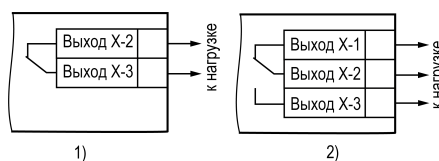
Рисунок 5.14 – Подключение нагрузки к ВУ типа «Р»: 1) к выходам 1 ...4, 2) к выходам 5 ...8
