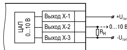
Рисунок 5.21 – Схема подключения нагрузки к ВУ типа «У»
