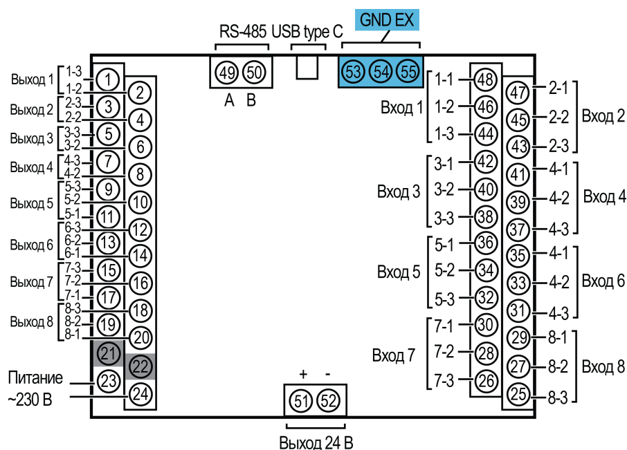
Рисунок 5.3 – Назначение контактов клеммника TPM138B
