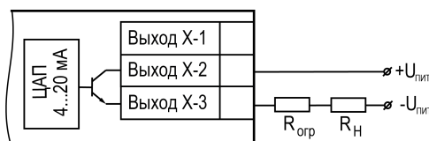
Рисунок 5.20 – Подключение к ВУ типа «И» с ограничивающим резистором
