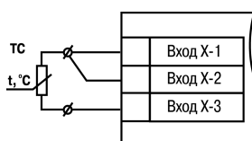
Рисунок 5.7 – Трехпроводная схема подключения ТС
