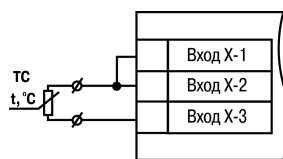
Рисунок 5.8 – Двухпроводная схема подключения ТС
