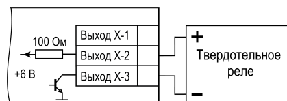
Рисунок 5.16 – Схема подключения нагрузки к ВУ типа «Т»
