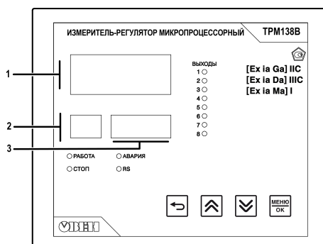
Рисунок 6.2 – Лицевая панель: 1) ЦИ–1, 2) ЦИ–2, 3) ЦИ–3
