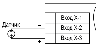
Рисунок 5.10 – Схема подключения активного датчика с выходом в виде сигнала напряжения постоянного тока от –50 до +50 мВ или от 0 до 1 В
