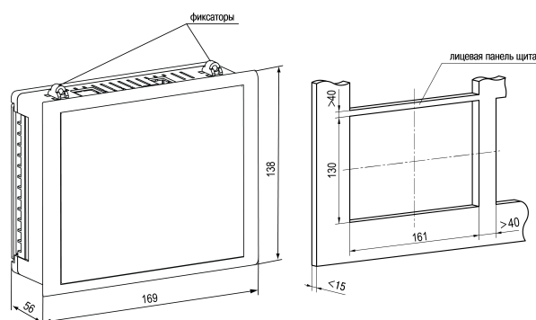
Рисунок 4.2 – Габаритные размеры корпуса Щ7
