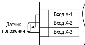
Рисунок 5.13 – Подключение датчика положения резистивного типа
