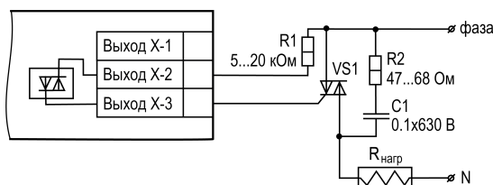
Рисунок 5.17 – Схема подключения силового симистора к ВУ типа «С»
