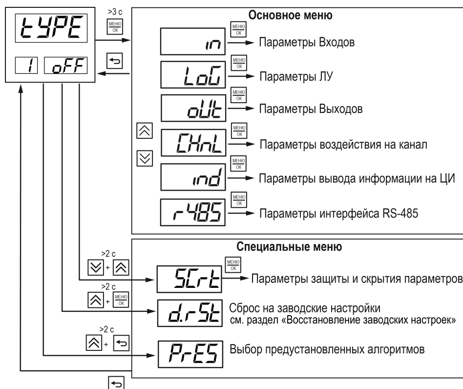
Рисунок 7.1 – Структура меню
