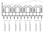
Рисунок 12 – Схема подключения к выходам типа «Р»
