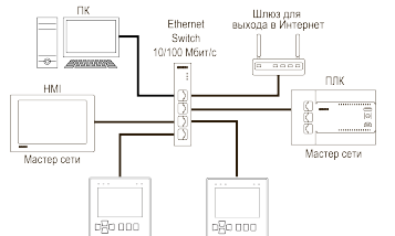
Рисунок 15 – Подключение по схеме «Звезда»
