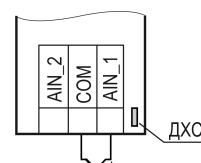
Рисунок 7 – Подключение ТП
