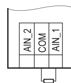
Рисунок 8 – Подключение резистивных датчиков по двухпроводной схеме
