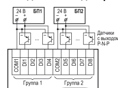
Рисунок 3 – Схема подключения к дискретным входам трехпроводных датчиков, имеющих выходной транзистор р-п-р-типа с открытым коллектором для сигналов 24 В
