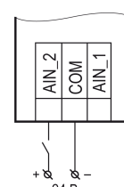
Рисунок 5 – Подключение дискретных датчиков к универсальным входам типа "TRM"
