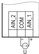
Рисунок 9 – Схема подключения датчиков с выходными сигналами постоянного напряжения от -50 до +50 мВ
