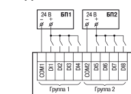
Рисунок 4 – Схема подключения дискретных датчиков с питанием 24 В к входам типа «Д»
