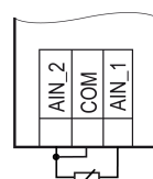
Рисунок 6 – Подключение ТС и других резистивных датчиков по трехпроводной схеме
