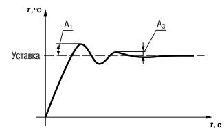
Рисунок Б.2 – График для определения ошибки регулирования
