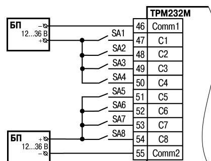
Рисунок 6.6 – Подключение датчиков к дискретным входам
