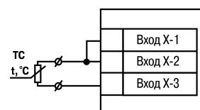
Рисунок 6.8 – Двухпроводная схема подключения ТС
