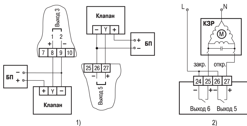
Рисунок 6.12 – Подключение клапана с аналоговым управлением к ВУ типа У (на примере подключения клапанов с приводами типа: 1) ST.0, 2) HR230–3)
