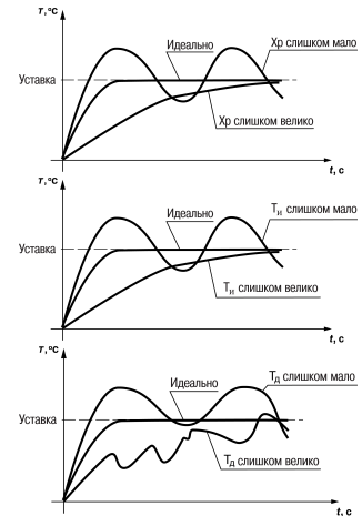
Рисунок Б.1 – Различные виды переходного процесса
