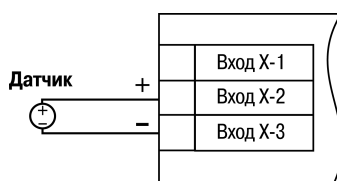
Рисунок 6.10 – Схема подключения активного датчика с выходом в виде напряжения или 0...1 В
