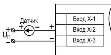
Рисунок 5.21 – Схема подключения пассивного датчика с выходным сигналом силы постоянного тока от 0 до 5 мА или от 0(4) до 20 мА
