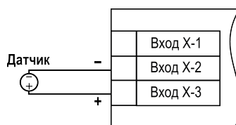
Рисунок 5.19 – Схема подключения активного датчика с выходными сигналами напряжения постоянного тока от -50 до +50 мВ или от 0 до 1 В
