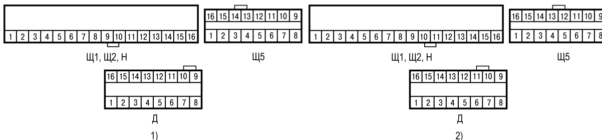
Рисунок 7.9 – Установка переключки
