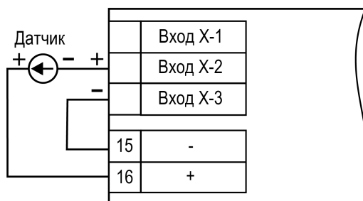
Рисунок 5.14 – Подключение токового датчика с питанием от ИП24
