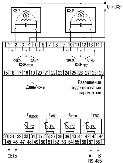
Рисунок В.2 – Схема подключения ТРМ32-Щ4
