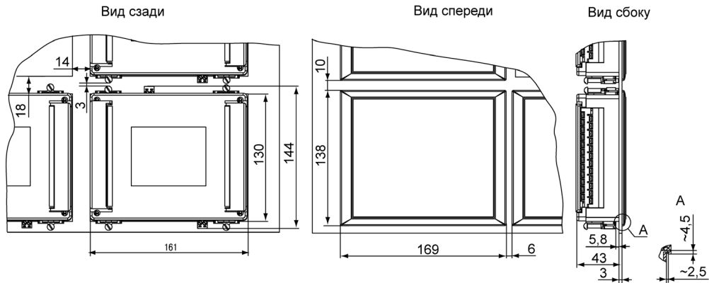
Рисунок Б.4 – Размеры TPM32-Щ7, установленного в щит толщиной 3 мм
