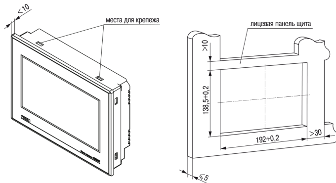
Рисунок 3 – Установочные размеры СП307
