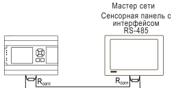
Рисунок 12 – Типовая схема подключения в режиме Slave
