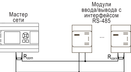
Рисунок 13 – Типовая схема подключения в режиме Master
