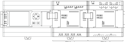
Рисунок 15 – Расположение модулей расширения на шине
