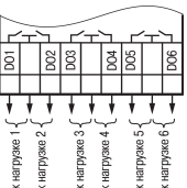
Рисунок 9 – Схема подключения ВЗ типа «Р»
