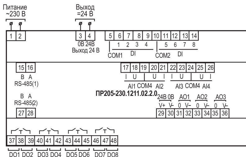
Рисунок А.2 – Расположение контактов для PR205-230.1211.02.2.0
