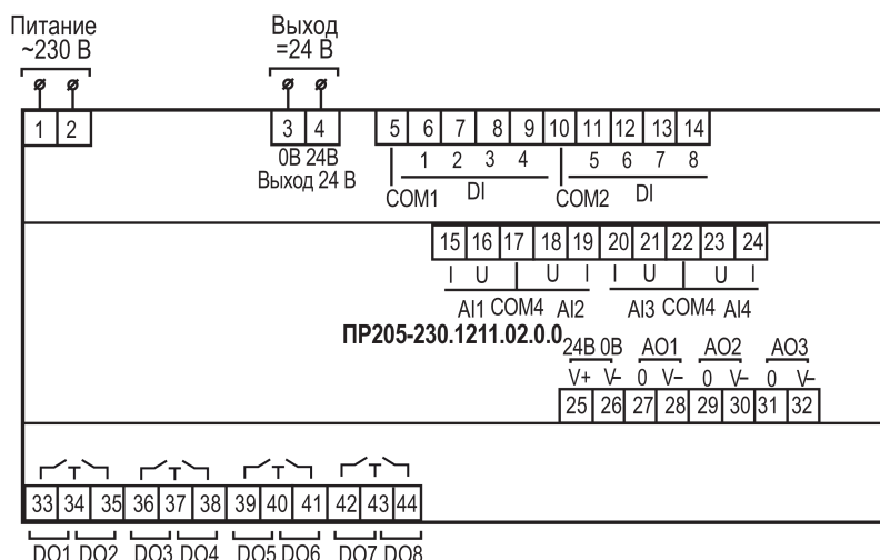
Рисунок А.1 – Расположение контактов для ПР205-230.1211.02.0.0
