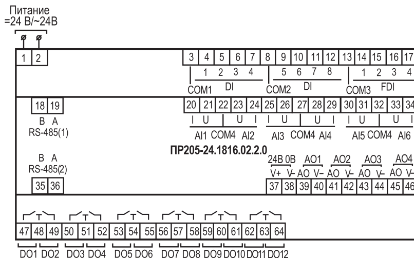
Рисунок А.18 – Расположение контактов для PR205-24.1816.02.2.0
