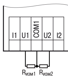
Рисунок 6.11 – Подключение резистивных датчиков
