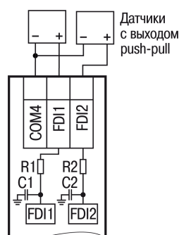
Рисунок 6.3 – Подключение к входам типа «ДС» датчиков с выходом push-pull
