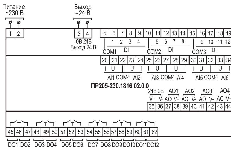
Рисунок А.9 – Расположение контактов для PR205-230.1816.02.0.0
