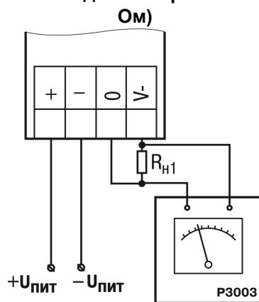
Рисунок В.4 – Схема подключения нагрузки к ВЭ для юстировки сигналов типа «0...10 В» ( R_H > 600 Ом)
