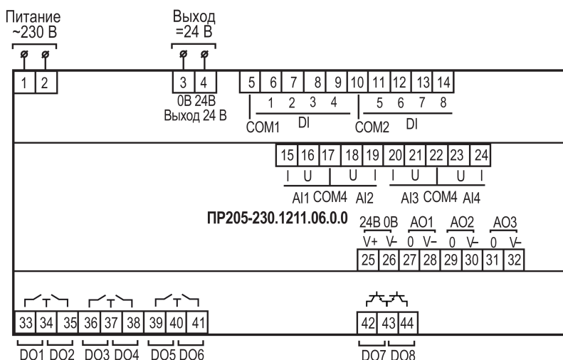
Рисунок А.3 – Расположение контактов для ПР205-230.1211.06.0.0
