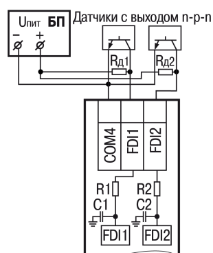
Рисунок 6.4 – Подключение к входам типа «ДС» датчиков с выходом n-p-n
