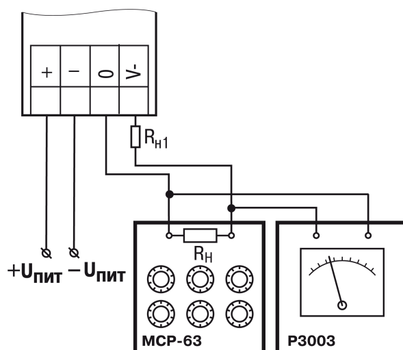
Рисунок В.3 – Схема подключения к ВЭ для юстировки сигналов типа «4...20 мА» ( R_H < 600
