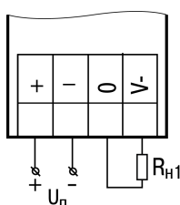
Рисунок 6.14 – Подключение аналогового выхода, находящегося в режиме источника тока
